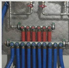
Коллекторная разводка труб водоснабжения
